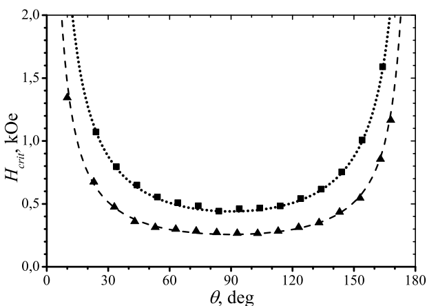
Рис. 3. Експериментально отримані залежності H_{crit}(\theta_H) для зовнішнього поля, що лежить у площині YZ ( \varphi_H = 90^\circ ) – ■ і XZ ( \varphi_H = 0 ) – ▲. Пунктирні лінії – апроксимація експериментальних залежностей H_{crit}(\theta_H) для \varphi_H = 90^\circ і \varphi_H = 0 виразами (17) і (18) відповідно
