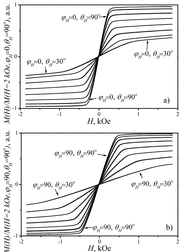
Рис. 2. Виділені гранулярні внески в петлі перемагнічування НГ плівки Co/Al_2O_n для різних кутів 30^\circ \leq \theta_H \leq 90^\circ : а – \mathbf{H} у площині XZ ; б – \mathbf{H} у площині YZ
