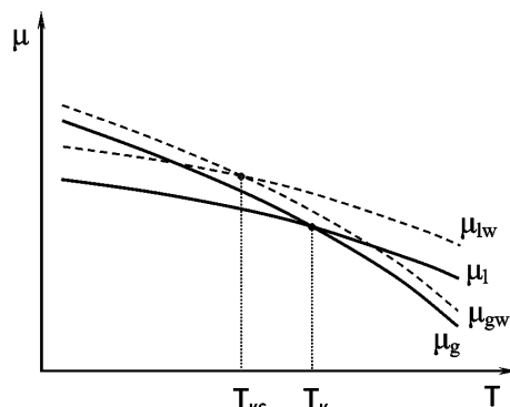
Рис. 1. Залежність хімічних потенціалів газу \mu_g , газу за наявності гідрофобної стінки, рідини \mu_l і рідини при наявності гідрофобної стінки ( [p = \text{const}] ): T_k – звичайна температура фазової рівноваги, T_{kc} – поблизу стінки
