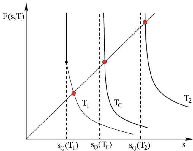
Рис. 3. Графічне розв'язання рівняння (6) в області крос-овера ( \mu \leq \mu_{сер} ), де КПН є від'ємним [23, 26] і тому F(z_Q, T, \mu) залишається скінченним лише за малих температур. Тоді простий полюс (6) завжди є найправішою сингулярністю ізобаричного розподілу
