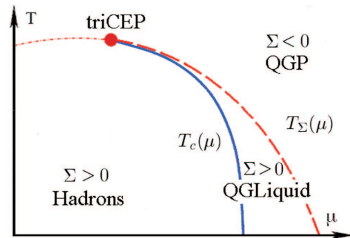
Рис. 4. Схематичне зображення фазової діаграми M1 у \mu-T координатах. КПН змінює знак вздовж пунктирної кривої T_\Sigma(\mu) . ФП деконфайнмента відбувається вздовж суцільної кривої T_c(\mu) при \mu > \mu_{сер} . При \mu < \mu_{сер} він вироджується в крос-овер (коротко-пунктирна крива T_\Sigma(\mu) ). Ці регіони відділені ТКТ, що позначена суцільним кругом
