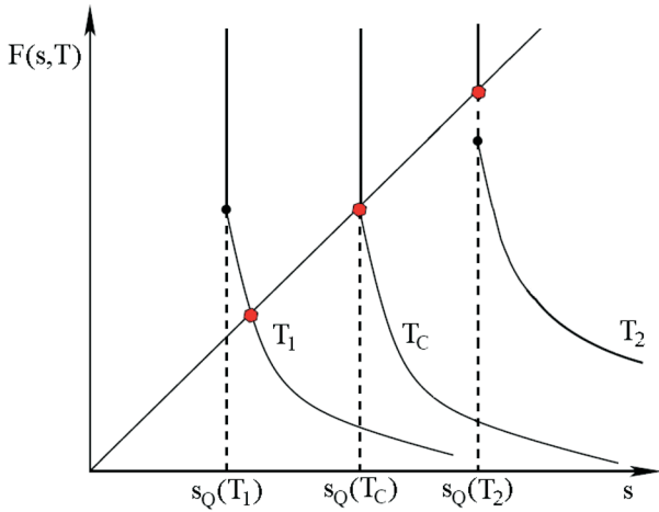
Рис. 1. Графічне розв'язання рівняння (6) в області ФП ( \mu > \mu_{\text{сер}} ) у випадку М1. Крива ФП лежить нижче кривої нульового значення КПН, тобто T_c(\mu) < T_\Sigma(\mu) , і тому F(z_Q, T, \mu) залишається скінченим при T < T_\Sigma(\mu) , де \Sigma > 0 . При малих температурах T_1 < T_c(\mu) простий полюс є найправішою сингулярністю \hat{Z}(T, \mu, z) і тому адронна фаза є домінуючою. За високих температур T_c(\mu) < T_2 < T_\Sigma(\mu) тиск системи визначається суттєво особливою сингулярністю (7), а отже фаза КГР є домінуючою. При критичному значенні температури T_c(\mu) відбувається ФП, за якого сингулярності (6) та (7) ізобаричного розподілу збігаються
