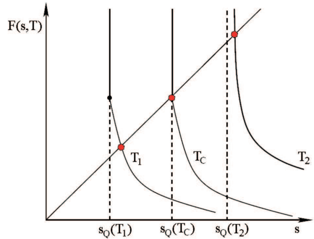
Рис. 2. Графічне розв'язання рівняння (6) в області ФП ( \mu > \mu_{\text{сер}} ) у випадку М2. Криві ФП та нульового значення КПН збігаються, тобто T_c(\mu) = T_\Sigma(\mu) , і тому F(z_Q, T, \mu) залишається скінченим при T < T_c(\mu) , де \Sigma > 0 . При малих T_1 < T_c(\mu) та великих T_2 > T_c(\mu) температурах простий полюс є найправішою сингулярністю \hat{Z}(T, \mu, z) і тому адронна фаза є домінуючою. КГР існує лише, коли сингулярності (6) та (7) ізобаричного розподілу збігаються під час ФП при температурі T_c(\mu)
