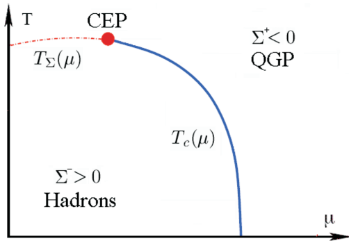
Рис. 5. Схематичне зображення фазової діаграми M2 у \mu - T координатах. ФП деконфайнмента відбувається вздовж суцільної кривої T_c(\mu) при \mu > \mu_{\text{сер}} . При \mu < \mu_{\text{сер}} він вироджується в крос-овер (пунктирна крива T_\Sigma(\mu) ). При \mu більших за критичне значення \mu_{\text{сер}} КПП змінює знак точно на кривій фазової рівноваги, тобто T_\Sigma(\mu) = T_c(\mu) при \mu > \mu_{\text{сер}} . Регіони ФП та крос-овера відділені КТ, що позначена суцільним кругом
