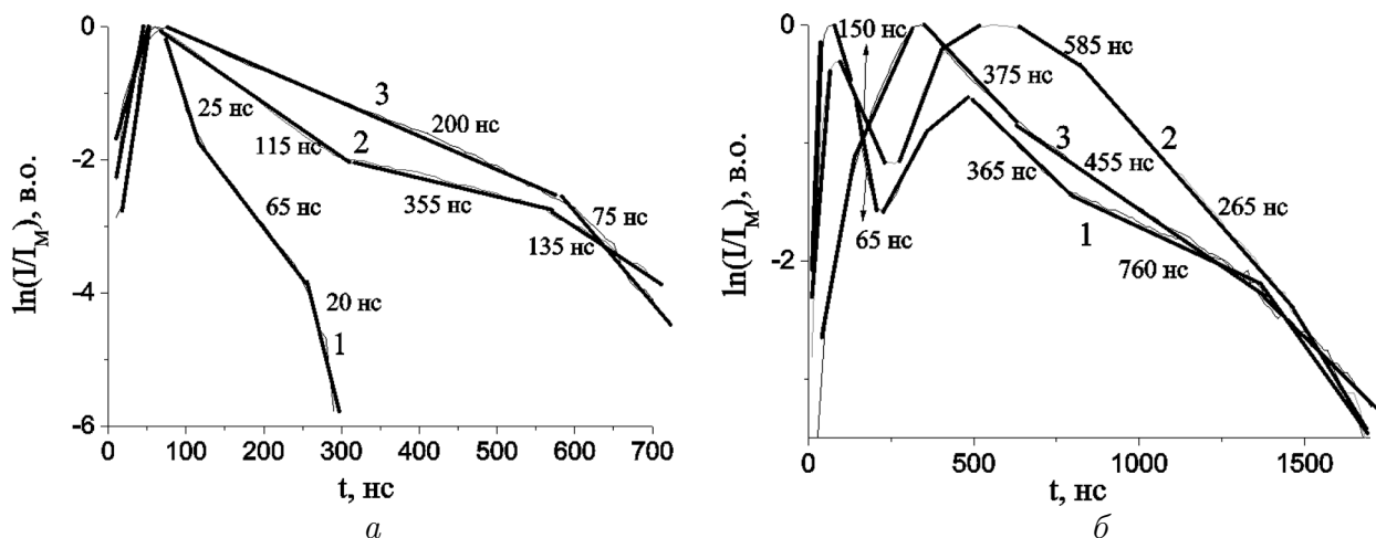
Рис. 3. Залежності логарифмів нормованих інтенсивностей спектральних ліній атомів та іонів олова від часу: 1 – 328,3 нм Sn II, E_B = 11,07 еВ; 2 – 242,9 нм Sn I, E_B = 5,52 еВ, 3 – 303,4 нм Sn I, E_B = 4,29 еВ на відстанях 1 мм (а) та 7 мм (б) від мішені
