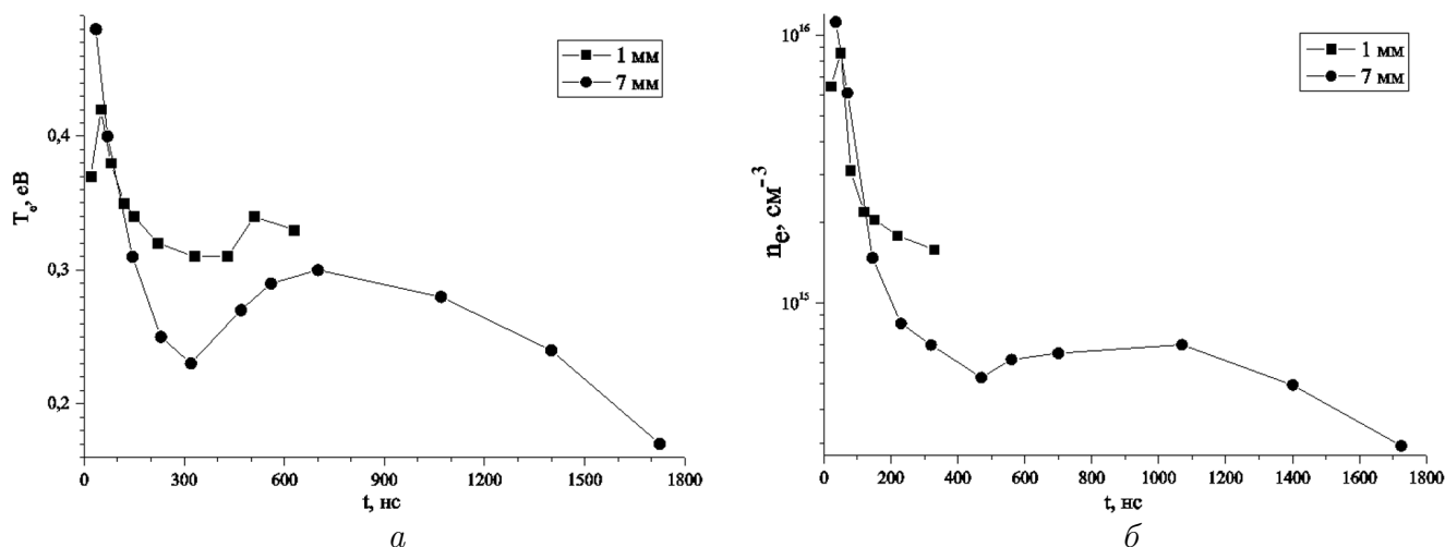
Рис. 2. Залежності температури (а) та концентрації (б) електронів від часу в лазерній плазмі олова
