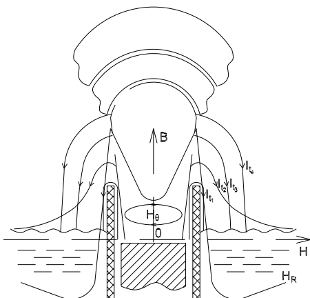
Рис. 2. Центральний електрод. Залізний струмовід у фарфоровому ізоляторі. Ізолятор на 1–5 мм виступає над рівнем електрода і води. Струмopровідний плазмoвий стовп і струмові канали – функції часу та відокремлені плазмoди. Радіальне магнітне поле та магнітні силові лінії усередині ізолятора
